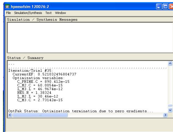
Fig. 15. Simulatorul ADS
